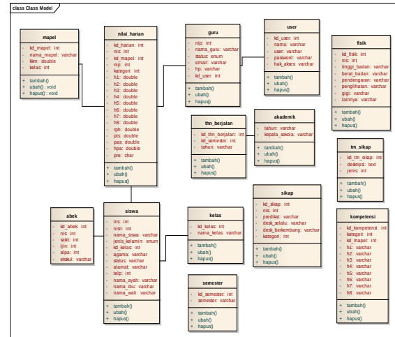
Gambar 8. Class Diagram Aplikasi Sistem Informasi Raport Online
